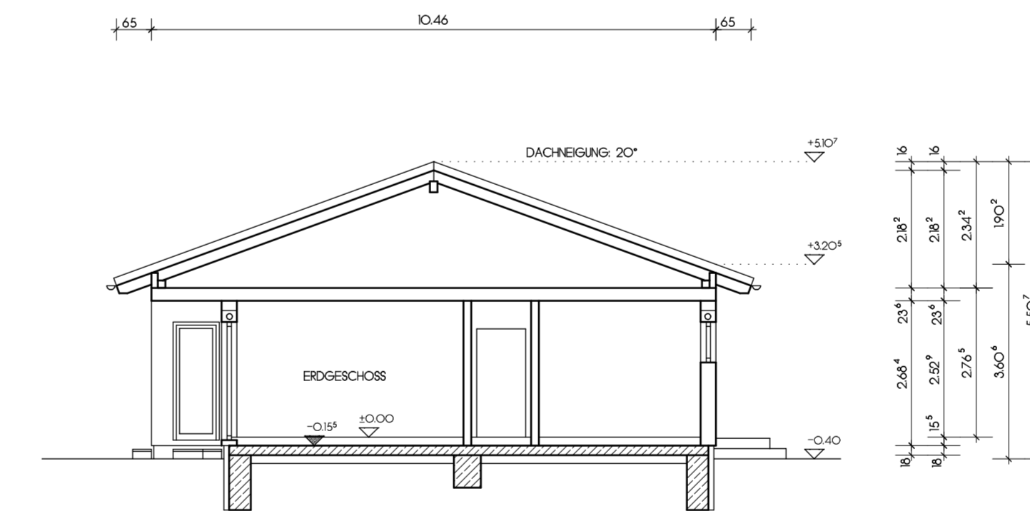
SCHNITT A-A
