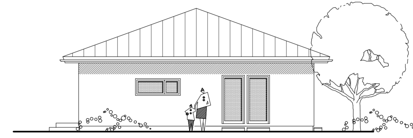
ANSICHT 1
