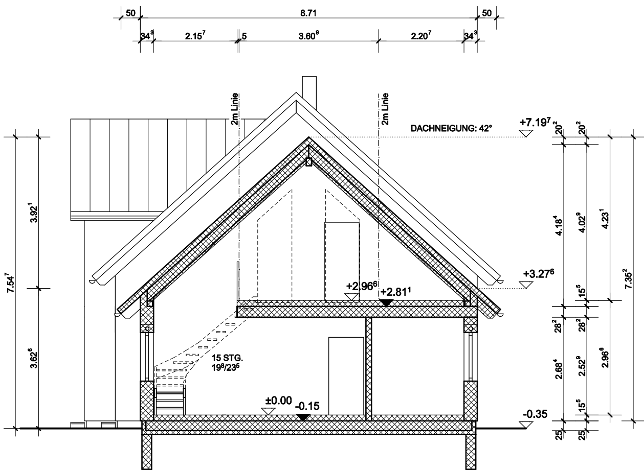
SCHNITT C-C
