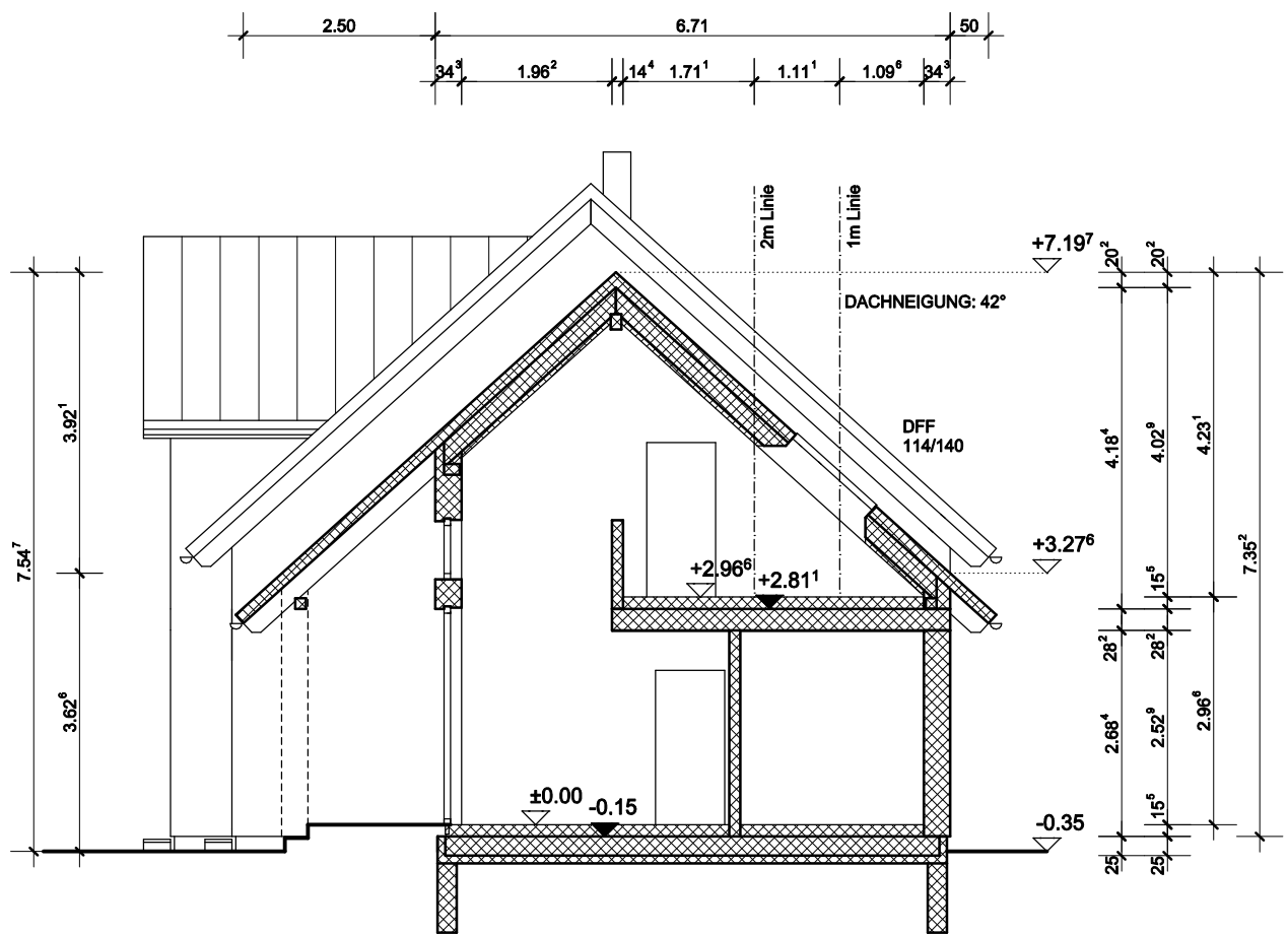
SCHNITT B-B
