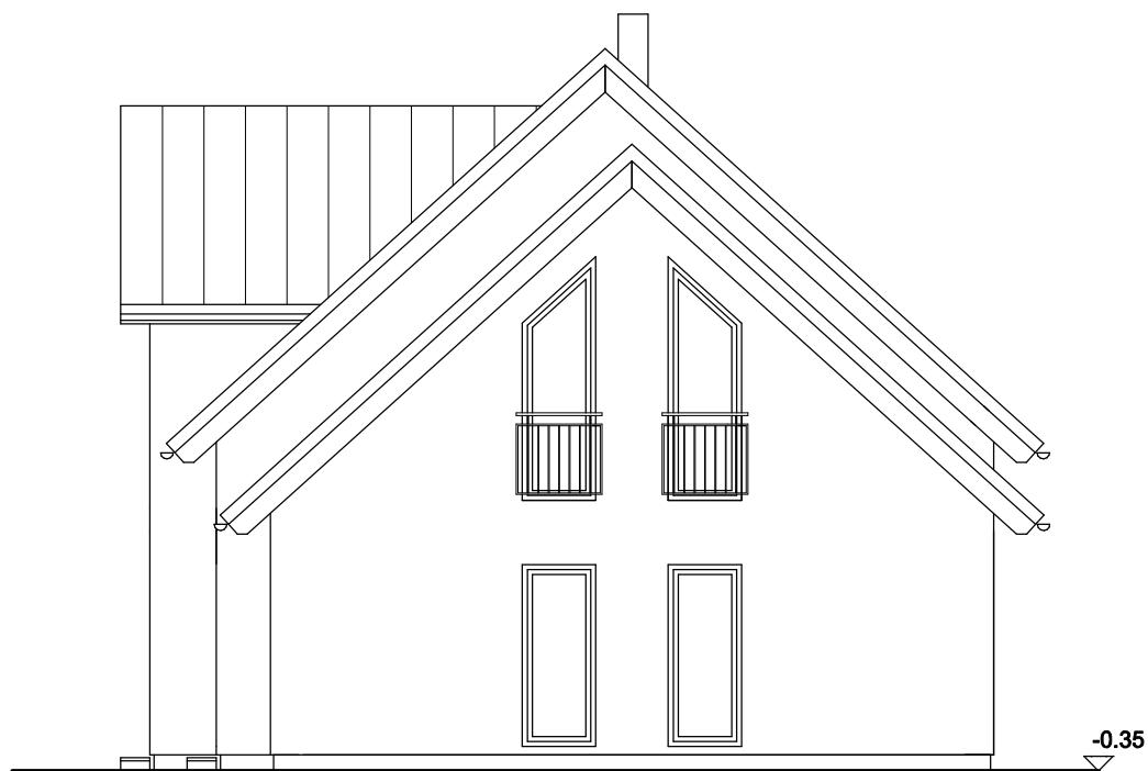
OSTANSICHT
