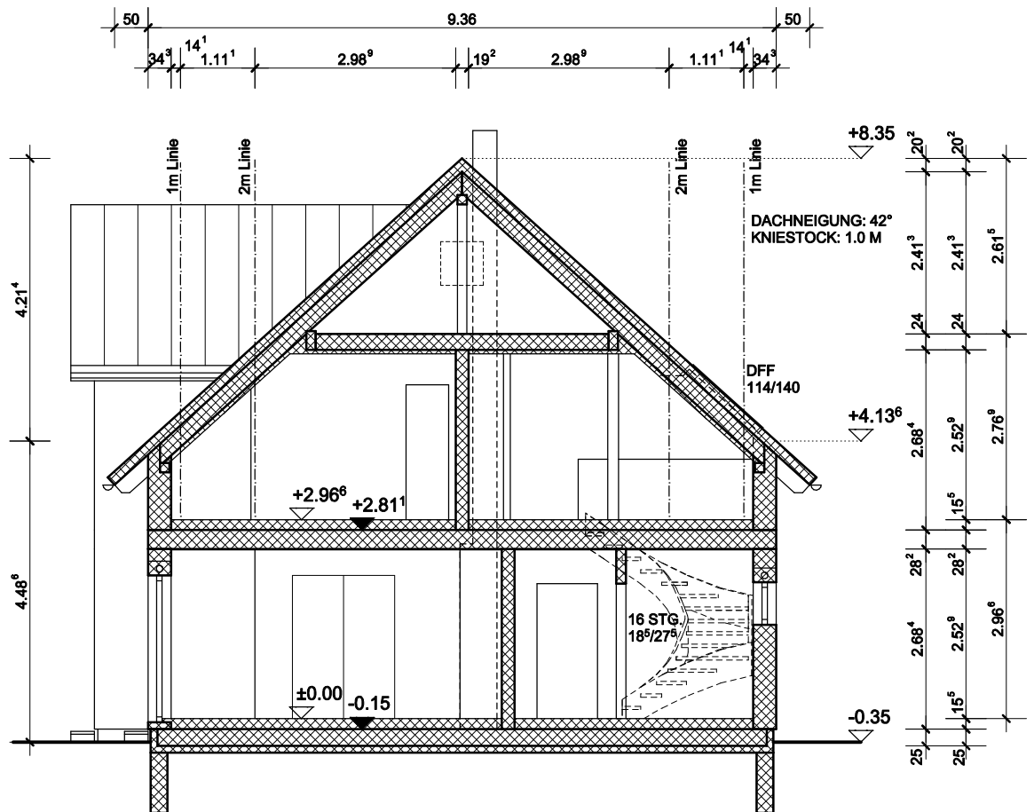
SCHNITT A-A
