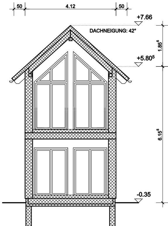
SCHNITT QUERGIEBEL
