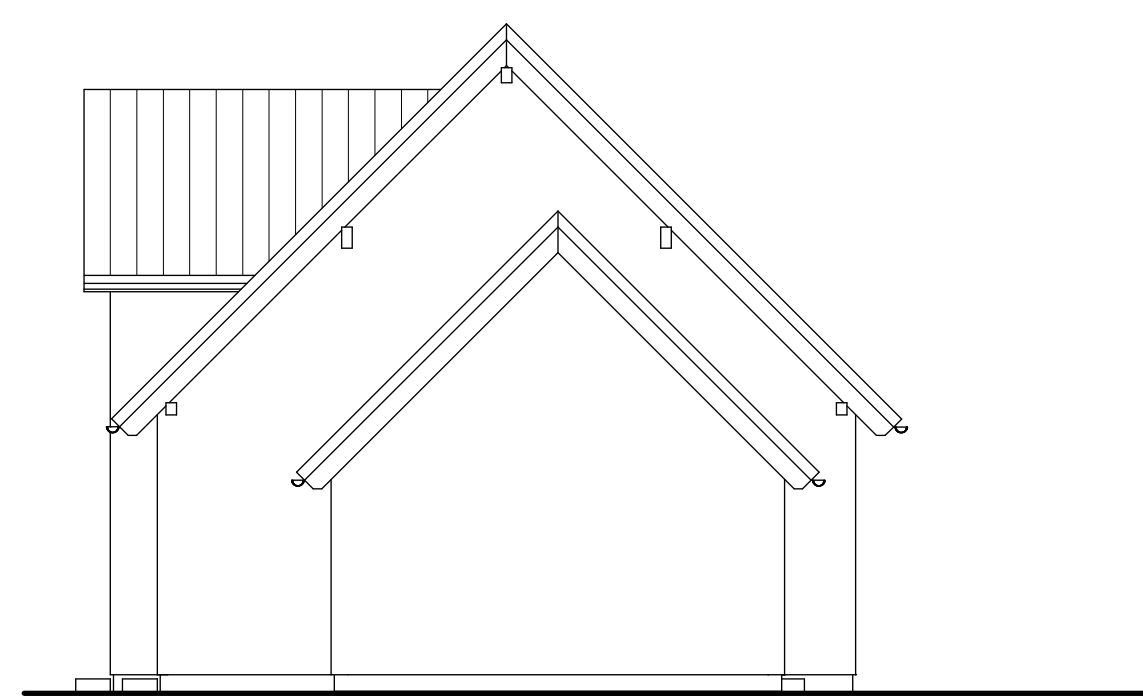
OSTANSICHT
