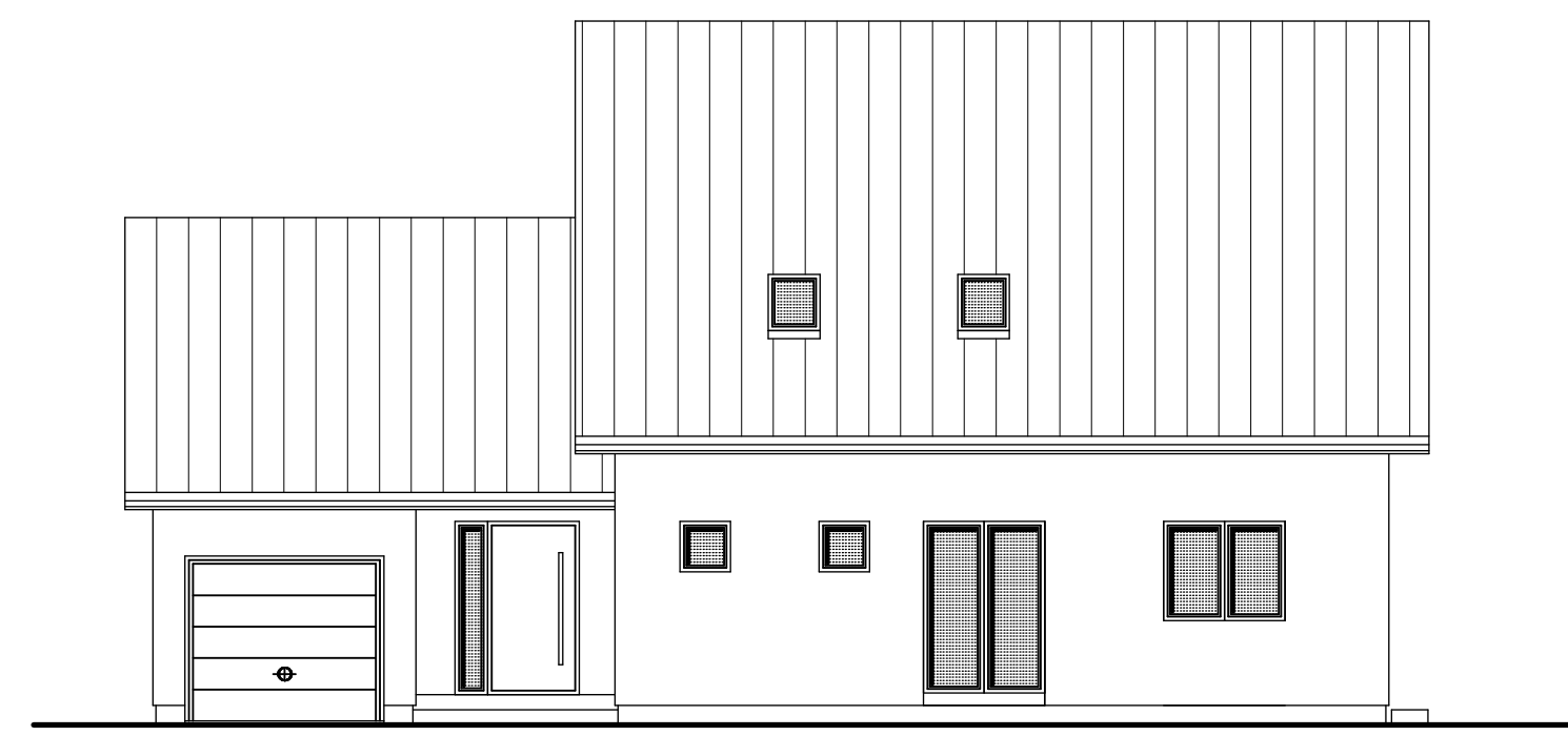
NORDANSICHT
