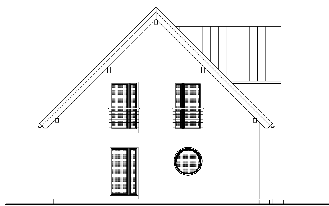
WESTANSICHT
