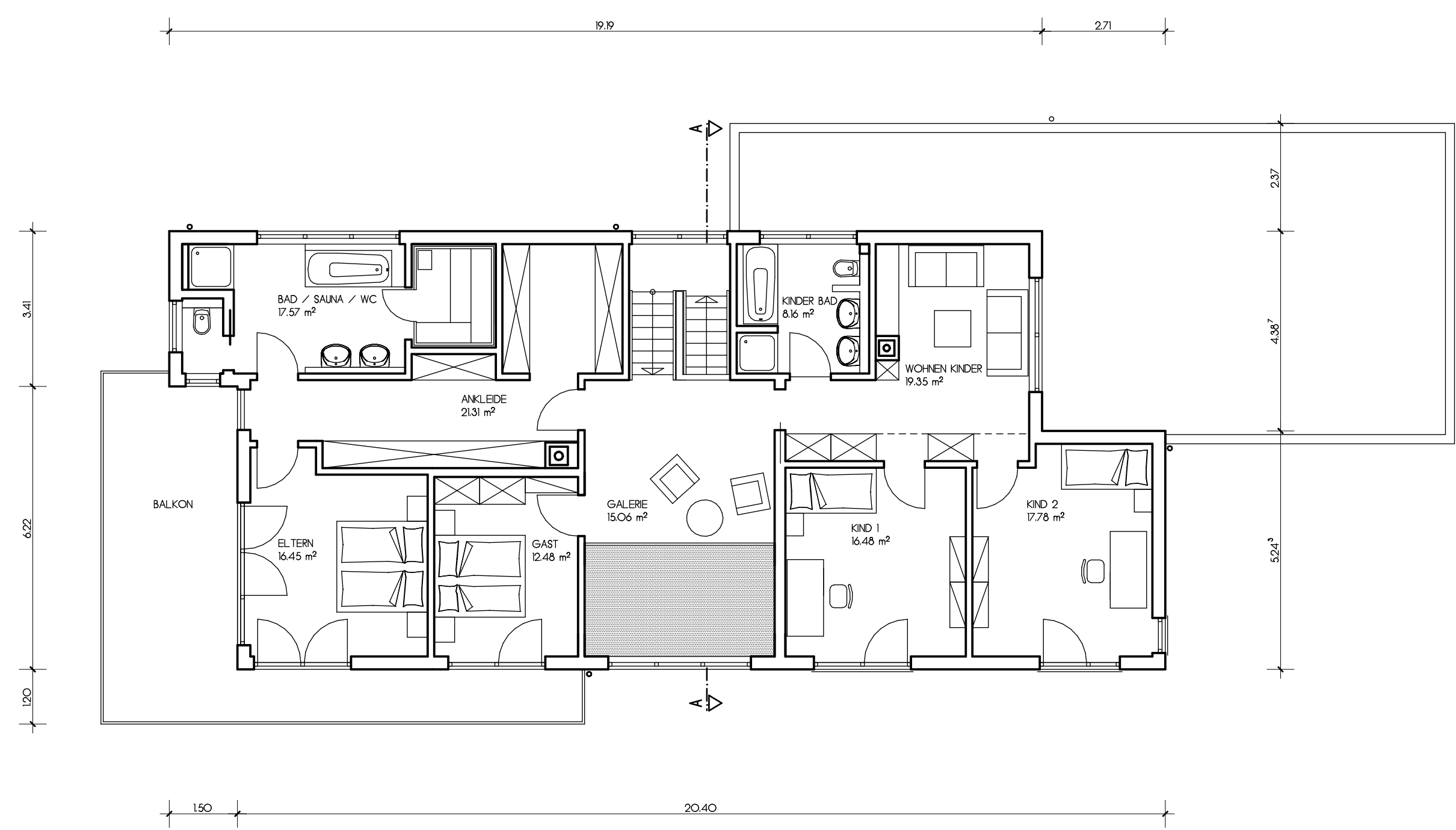
OBERGESCHOSS
