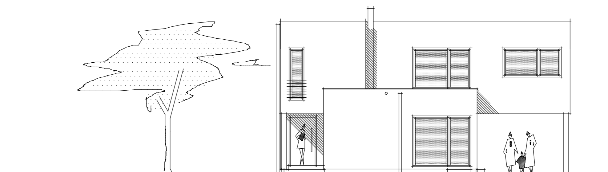
WESTANSICHT
