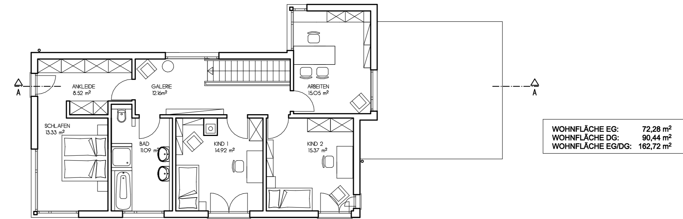
GRUNDRISS - OG
