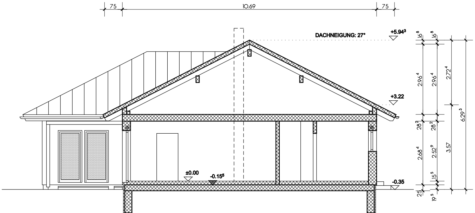
SCHNITT A-A
