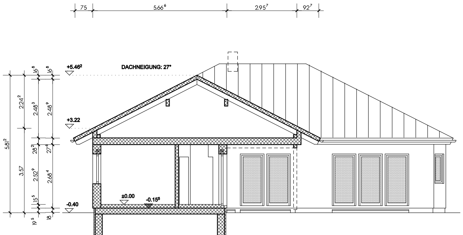
SCHNITT B-B
