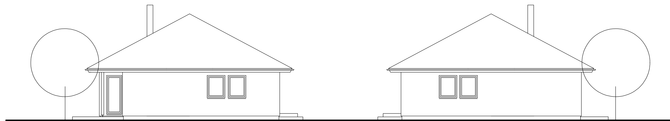
ANSICHT 1
