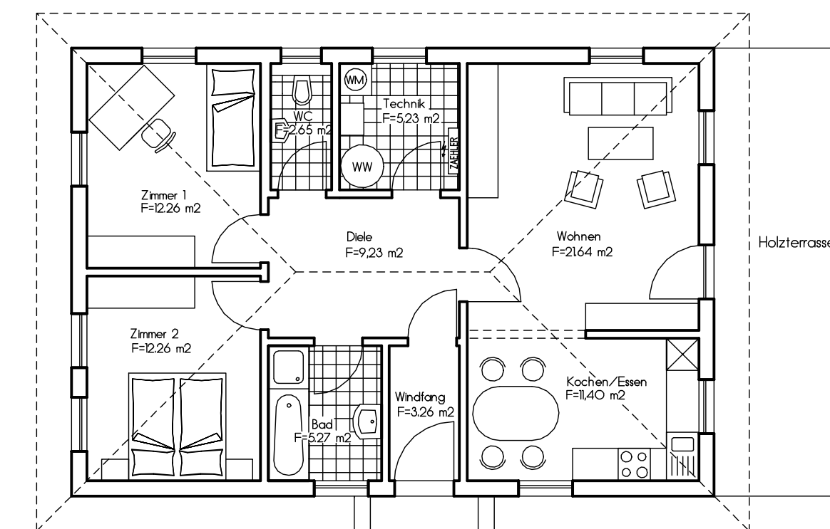
EG-GRUNDRISS VARIANTE MIT BODENPLATTE
