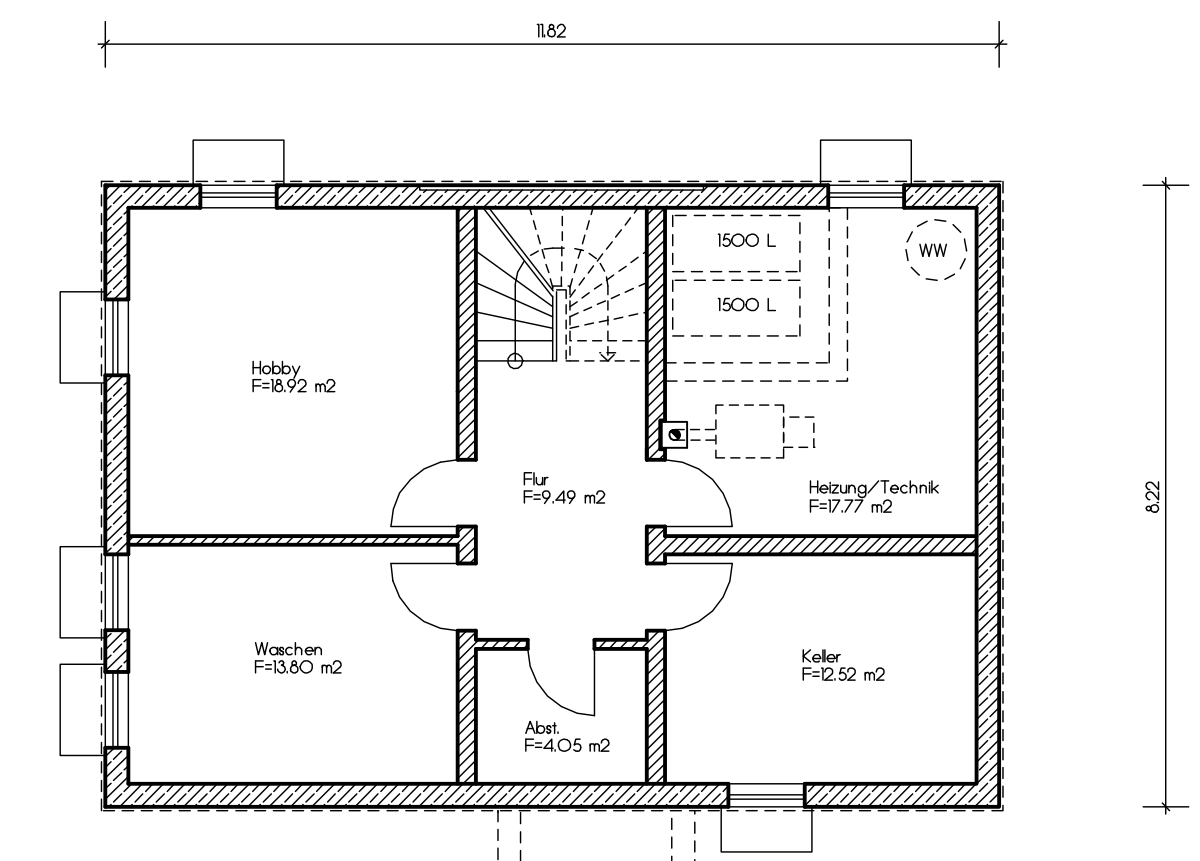
KG-GRUNDRISS KG-VORSCHLAG
