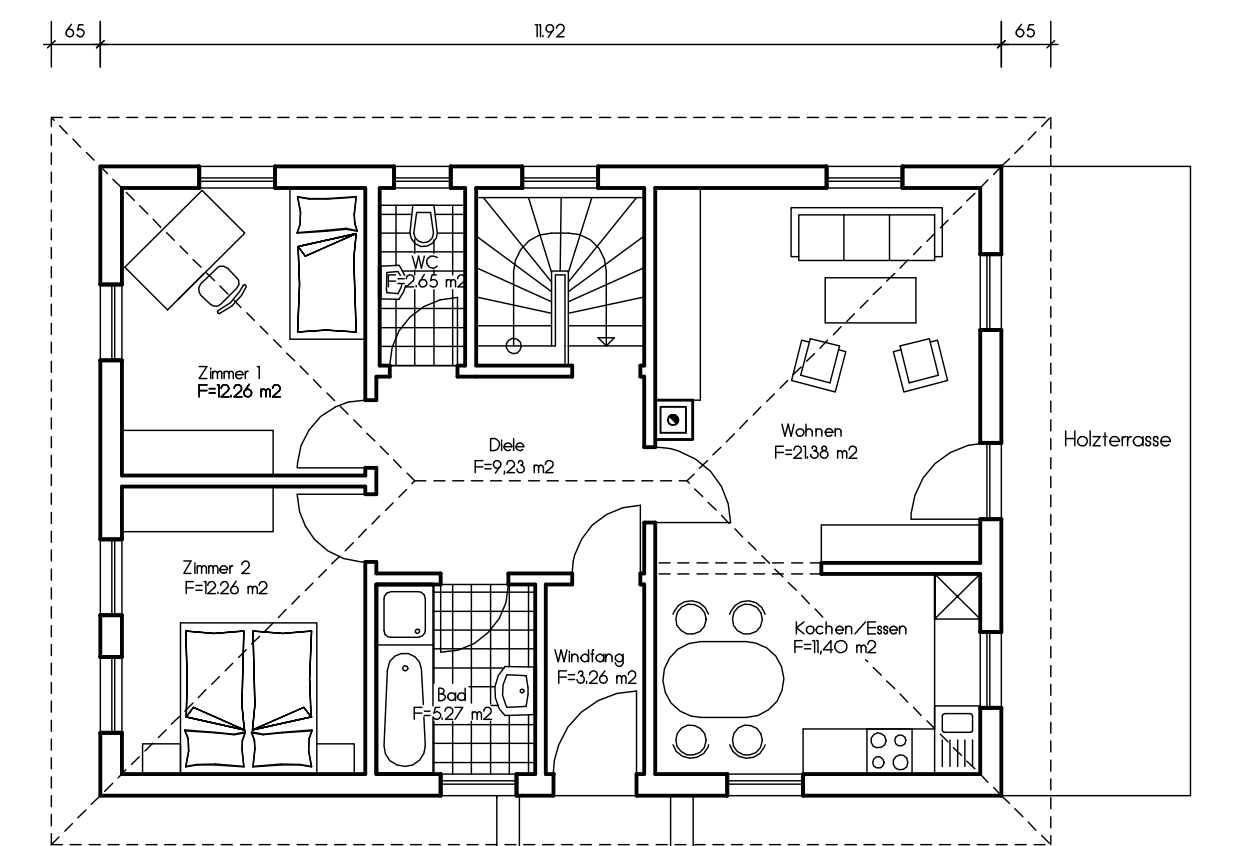
EG-GRUNDRISS VARIANTE MIT KELLER
